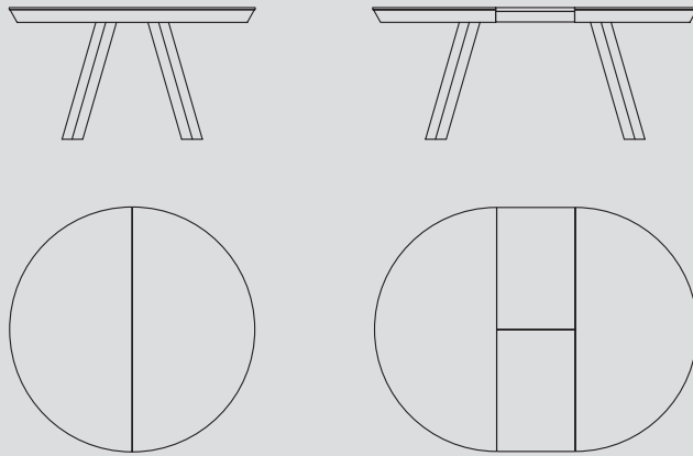
Ref. 5010 Ø125 (165x125) · Ø140 (185x140) · Ø150 (200x150)
